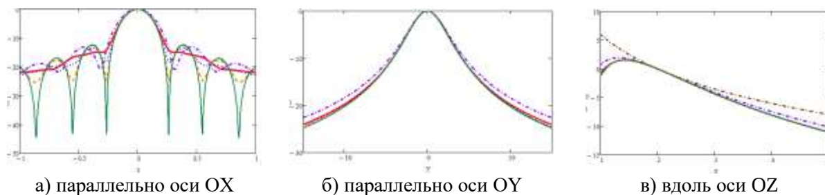
Рис. 5. Нормированные осевые распределения энергии электромагнитного поля, сфокусированного в зоне ближнего излученного поля с непрерывным спектром шириной 1000 МГц
