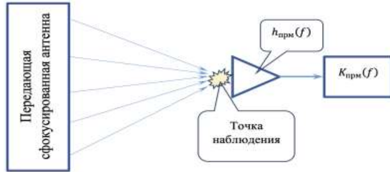
Рис. 1. Широкополосная сфокусированная антенна в режиме передачи
