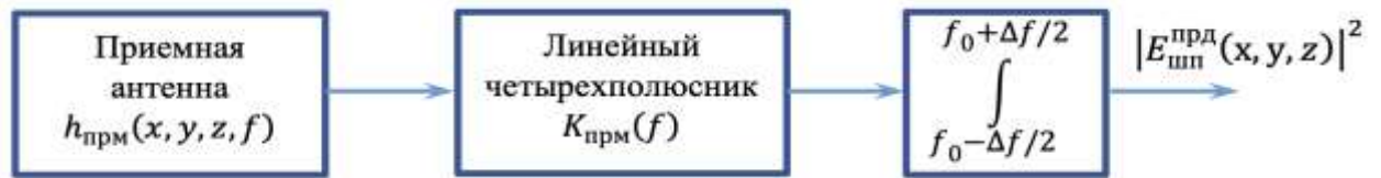
Рис. 2. Структурная схема приемной части
