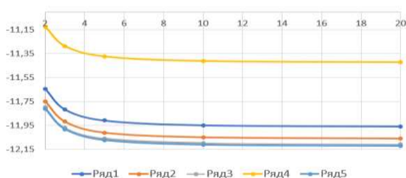
Рис. 6. Зависимость K_{скр} линейной СФДА от расстояния до точки фокусировки
