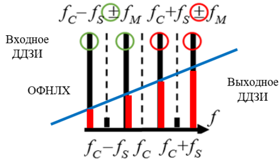
Рис. 3. Спектрограммы ДДЗИ на входе и выходе ОФНЛХ
