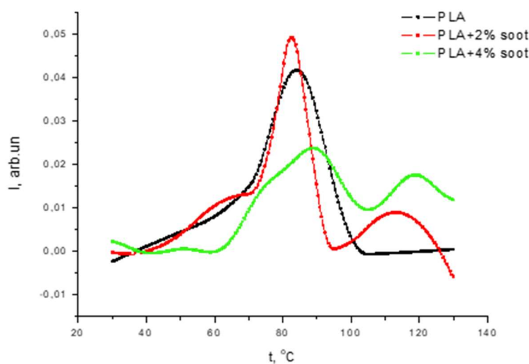
Рисунок 2. Температурные зависимости \frac{d\varphi}{dT} для пленок полилактида с различным процентным содержанием белой сажи
