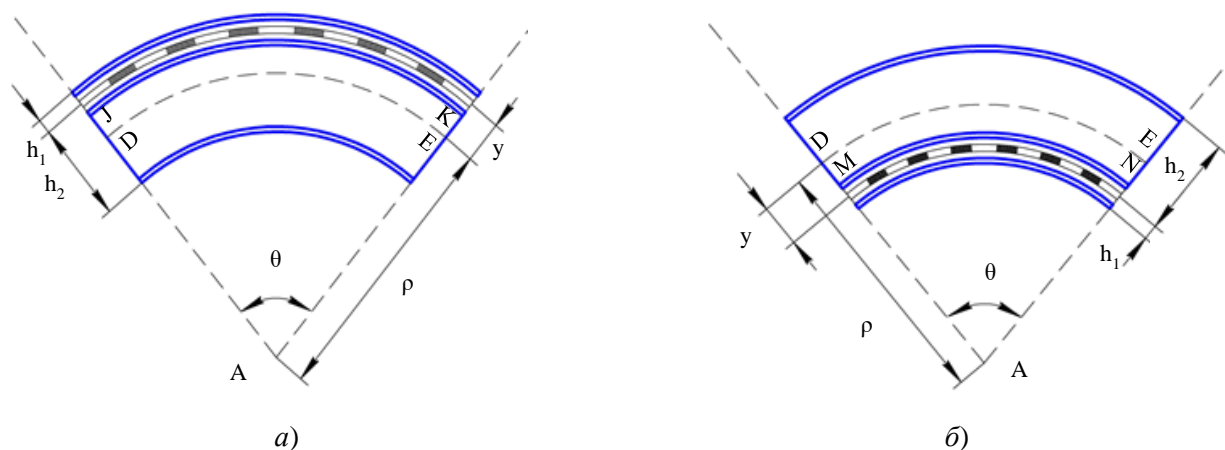
Рис. 1. К пояснению принципа работы диафрагмы: ситуация «положительного» изгиба для верхней поверхности с АВБС 1 (а); ситуация «отрицательного» изгиба» для нижней поверхности с АВБС 2 (б)
