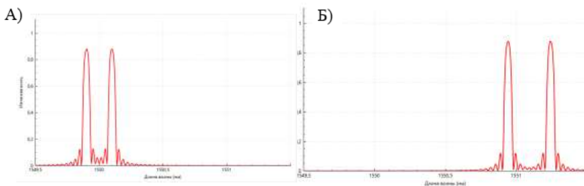
Рис. 2. Результаты моделирования базовой конфигурации: А) при 0 °C и 0 ppm; Б) при 100 °C и 500 ppm
