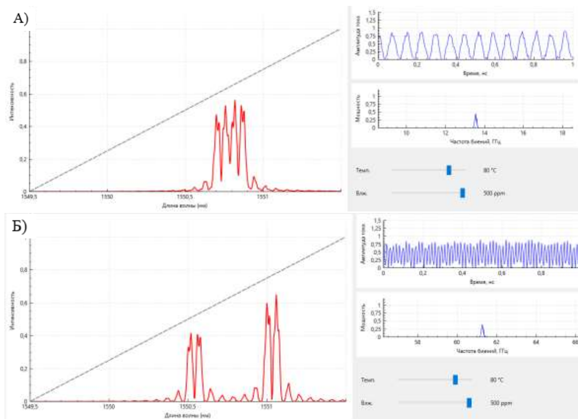
Рис. 4. Комплексное воздействие температуры и влажности на конфигурации:
